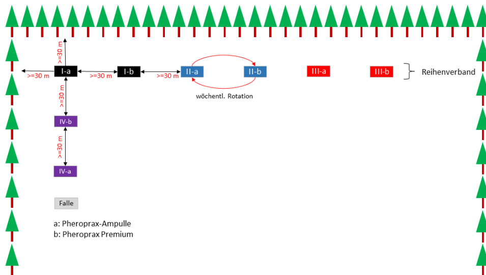
Abb. 7: Schematischer Aufbau des Vergleichsversuchs
